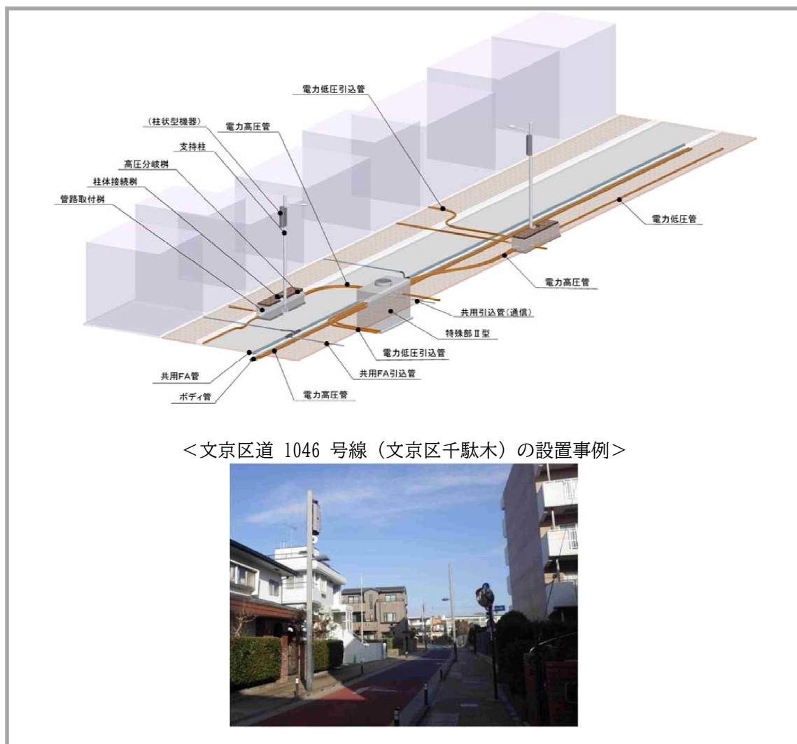
図 17 ソフト地中化のイメージ及び設置事例
