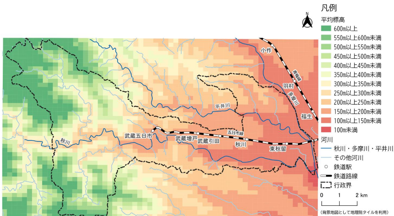
図 2-24 標高の状況※
