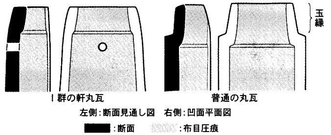
第2図 軒丸瓦の狭端部の模式図
