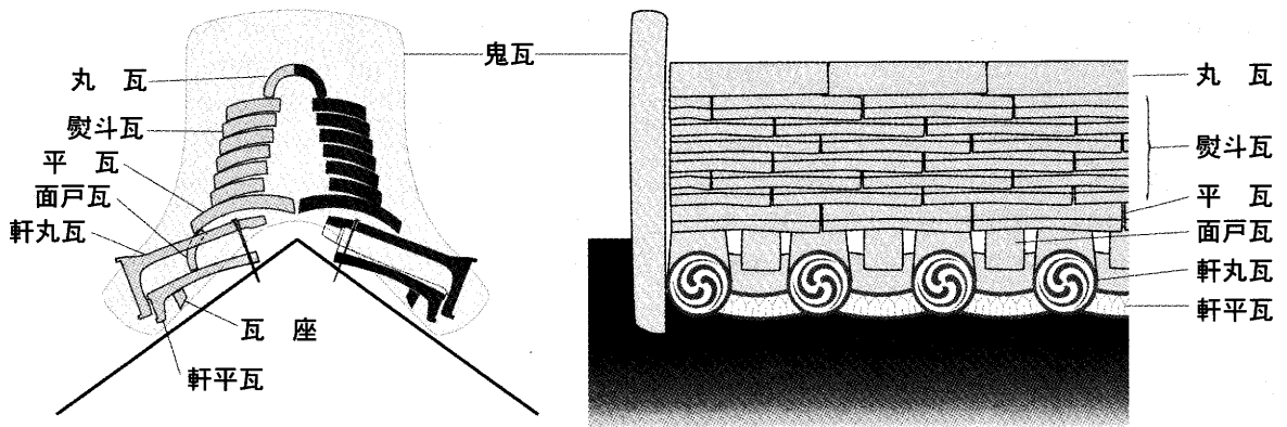
第3図 葺棟の推定復元図
